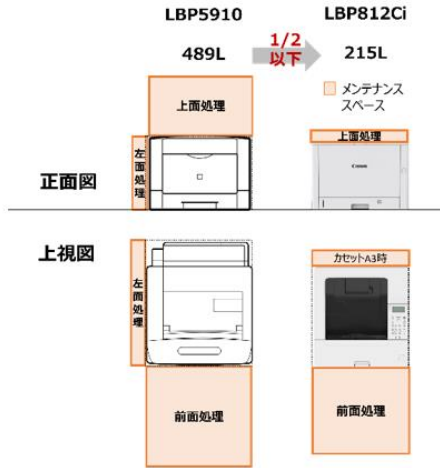
メンテナンスに必要な占有体積を大幅削減
